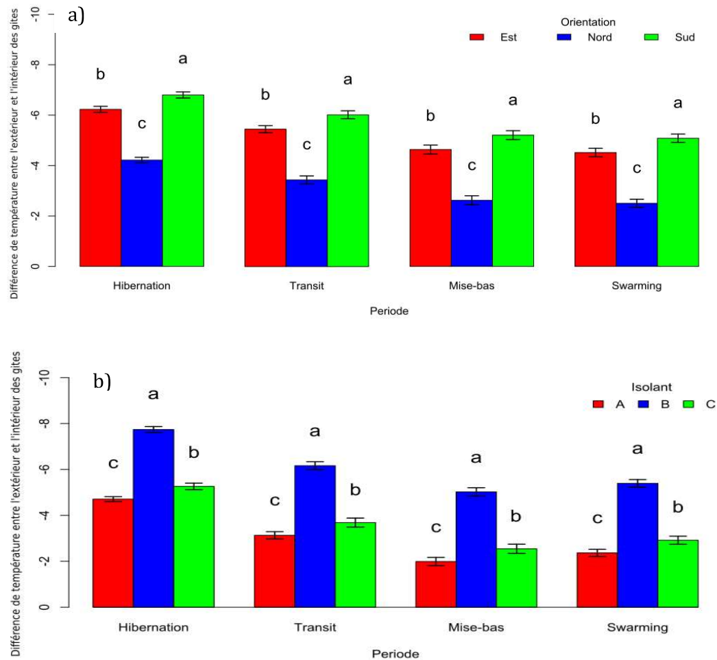
Figure 2 : Moyennes ajustées par le modèle des différences de températures horaires entre l'intérieur et l'extérieur des gîtes pour chacune des modalités des variables du modèle analysé par un test de Wald pour les variables : a) Orientation : Df=2 et p = < 2e-16 *** ; b) Isolation : Df=2 et p = 0.03196 * ; c) Aération : Df=1 et p = < 2e-16 *** en fonction de la période du cycle biologique (Df=3 et p = < 2e-16 *** ). Les lettres indiquent les
