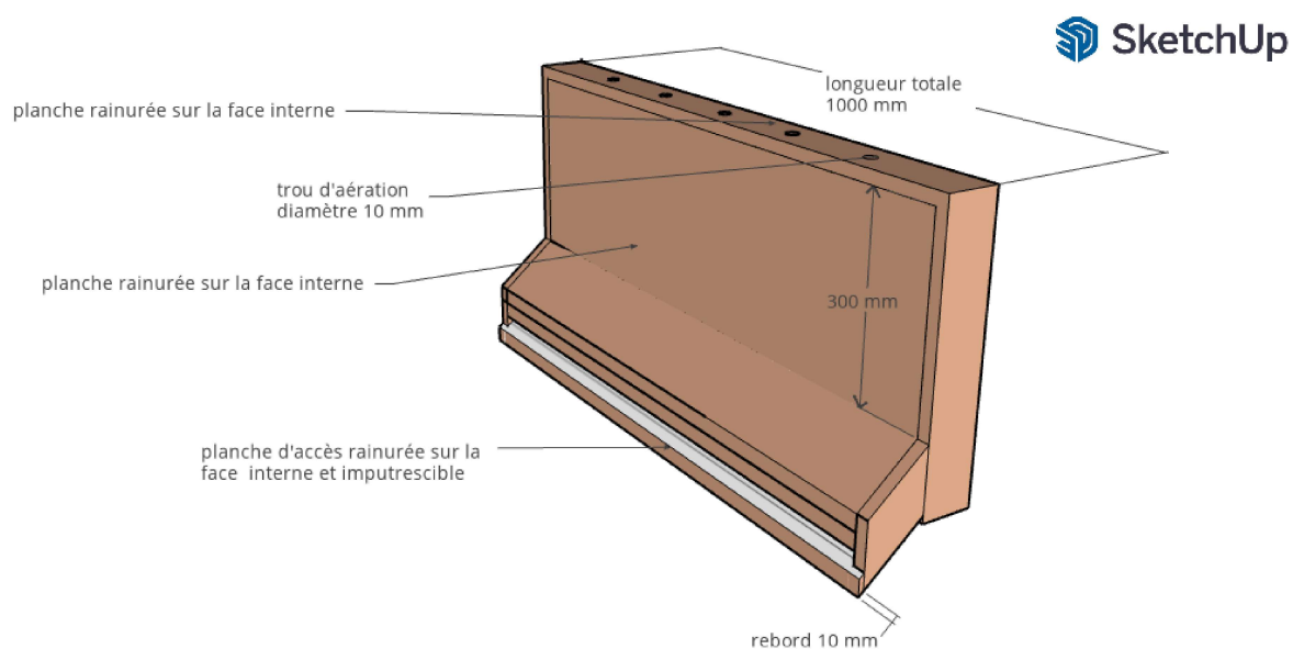
Figure 1 : Plan des gîtes installés dans les bâtiments, vue générale.
