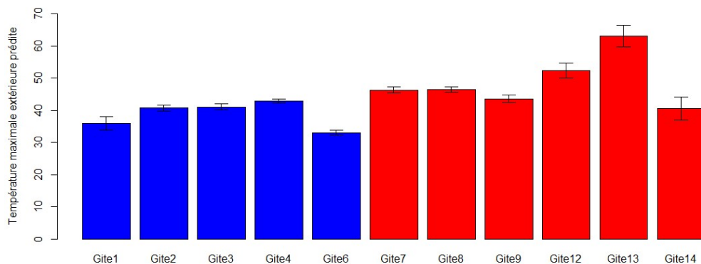
Figure 3 : Barplot représentant les températures extérieures prédites pour une température de 40°C à l'intérieur des gîtes. Les gîtes de l'IUT de Bourges apparaissent en bleu et les gîtes de la cité Didier Gerbaud de Saint-Amand-Montrond en rouge. Les barres d'erreurs correspondent à l'intervalle de confiance 0,95.
